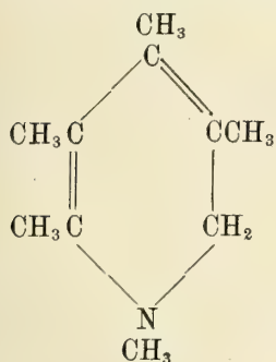
Pentametildiidropiridina
